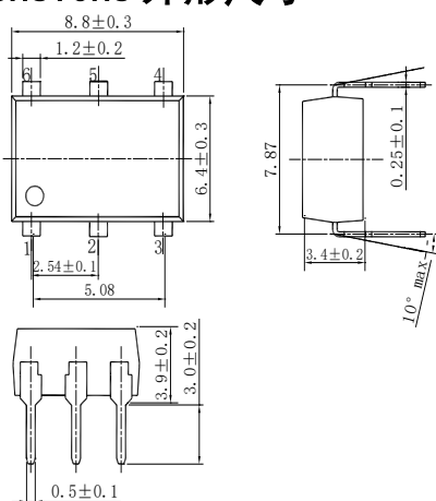
DIP6
