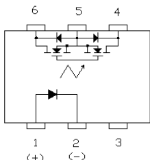
DIP6
