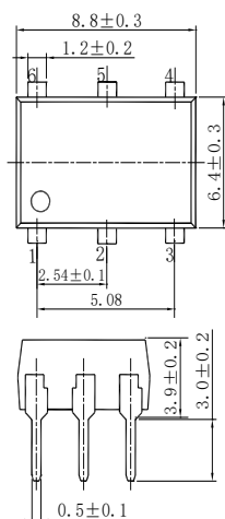
DIP6
